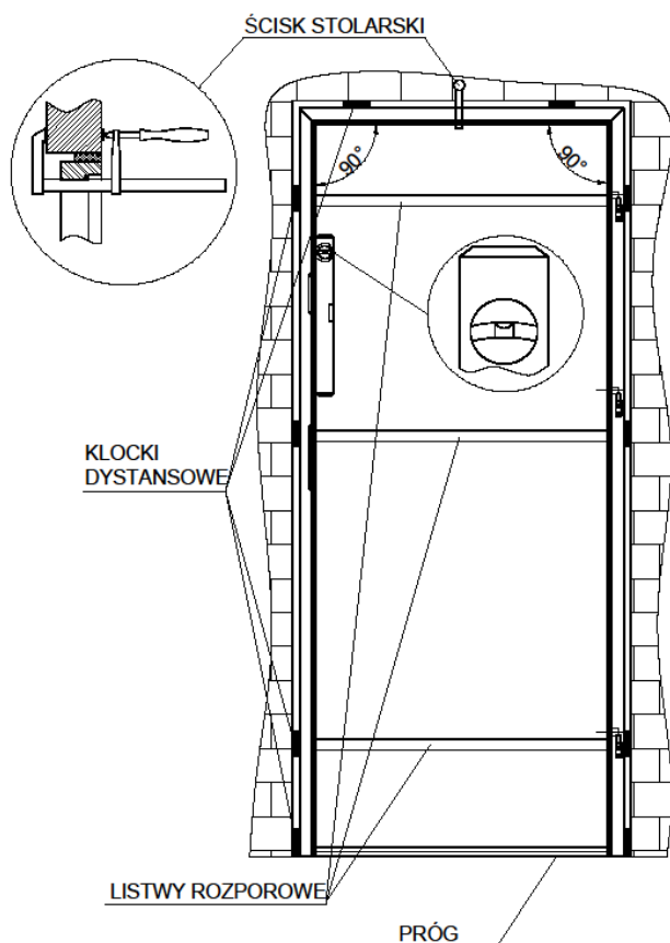
Rys. 1. Rozmieszczenie klocków dystansowych i listew rozporowych
