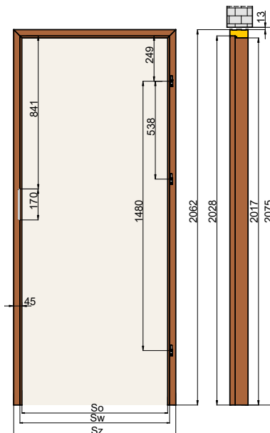
WYMIARY OŚCIEŻNIC STAŁYCH 100x45 mm DO DRZWI JEDNOSKRZYDŁOWYCH
